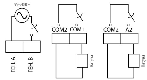
Подключение входа «Генератор / день-ночь»
