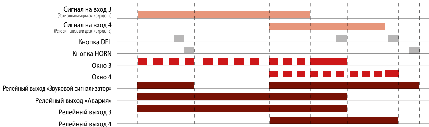
ВРЕМЕННЫЕ ДИАГРАММЫ
