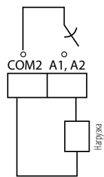
Подключение выхода реле сигнализации
